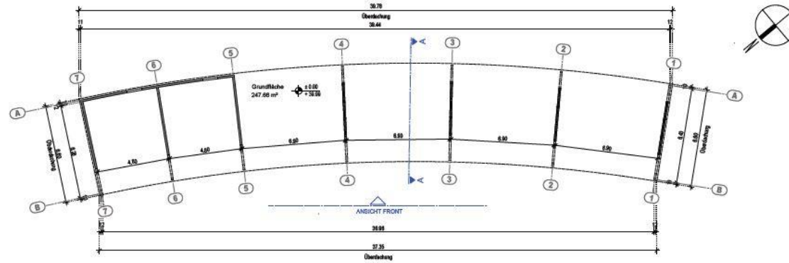
Grundriss M 1:200
